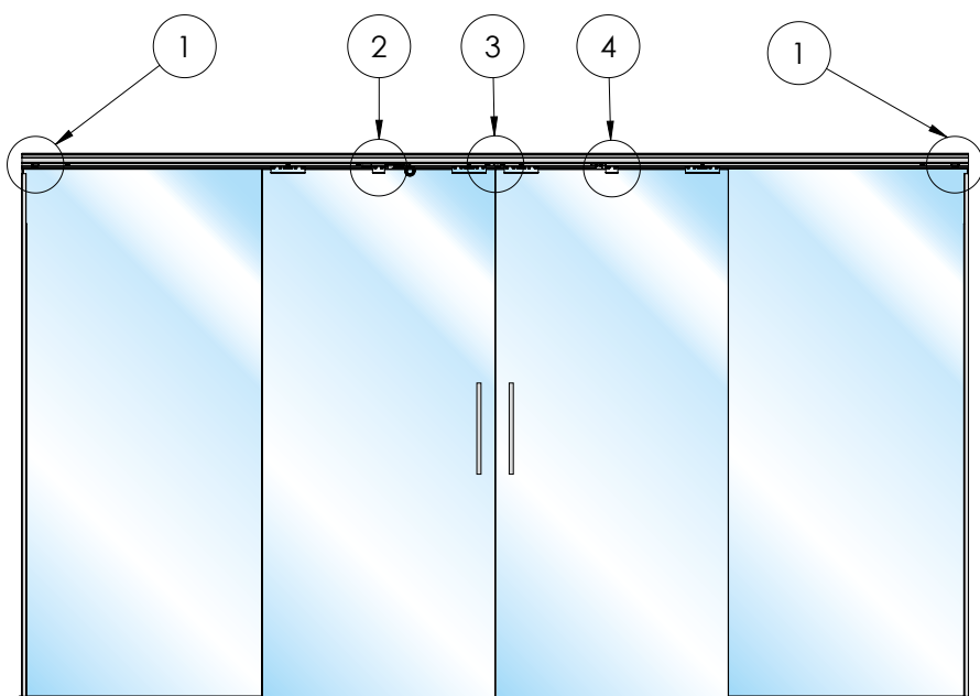
nr 91703000 samodomykacz SLX plus 40 kg soft-closer
